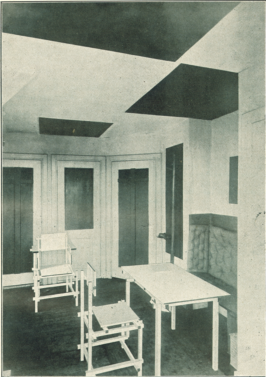
THEO VAN DOESBURG. PROEVE VAN KLEURENCOM- POSITIE IN INTÉRIEUR (1919). MEUBELN VAN G. RIET- VELD. BIJLAGE XIV VAN „DE STIJL” 3E JAARGANG No. 12.
