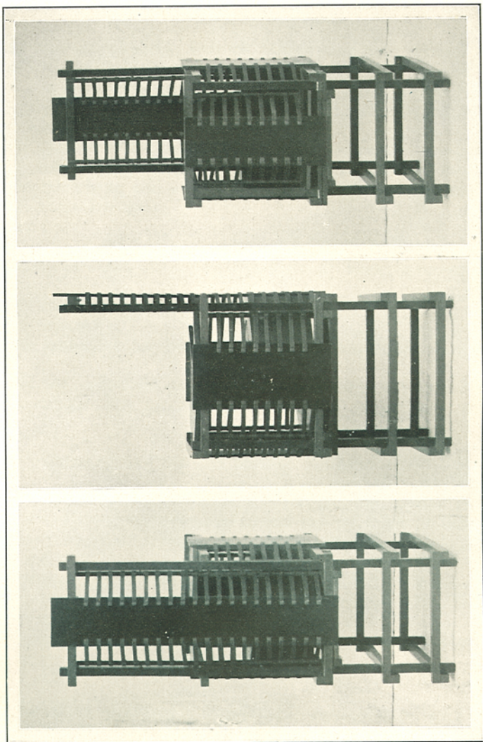
BIJLAGE XVIII VAN „DE STIJL”, 2E JAARGANG No. 9. VÓÓR-, OPZIJ- EN ACHTER- AANZICHT VAN EEN KINDERSTOEL. MAKER: RIETVELD.
