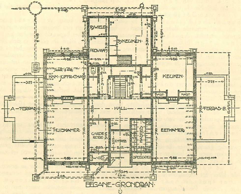
PLATTEGROND VACANTIEHUIS NOORDWIJKERHOUT (ZIE DE BIJLAGE).
